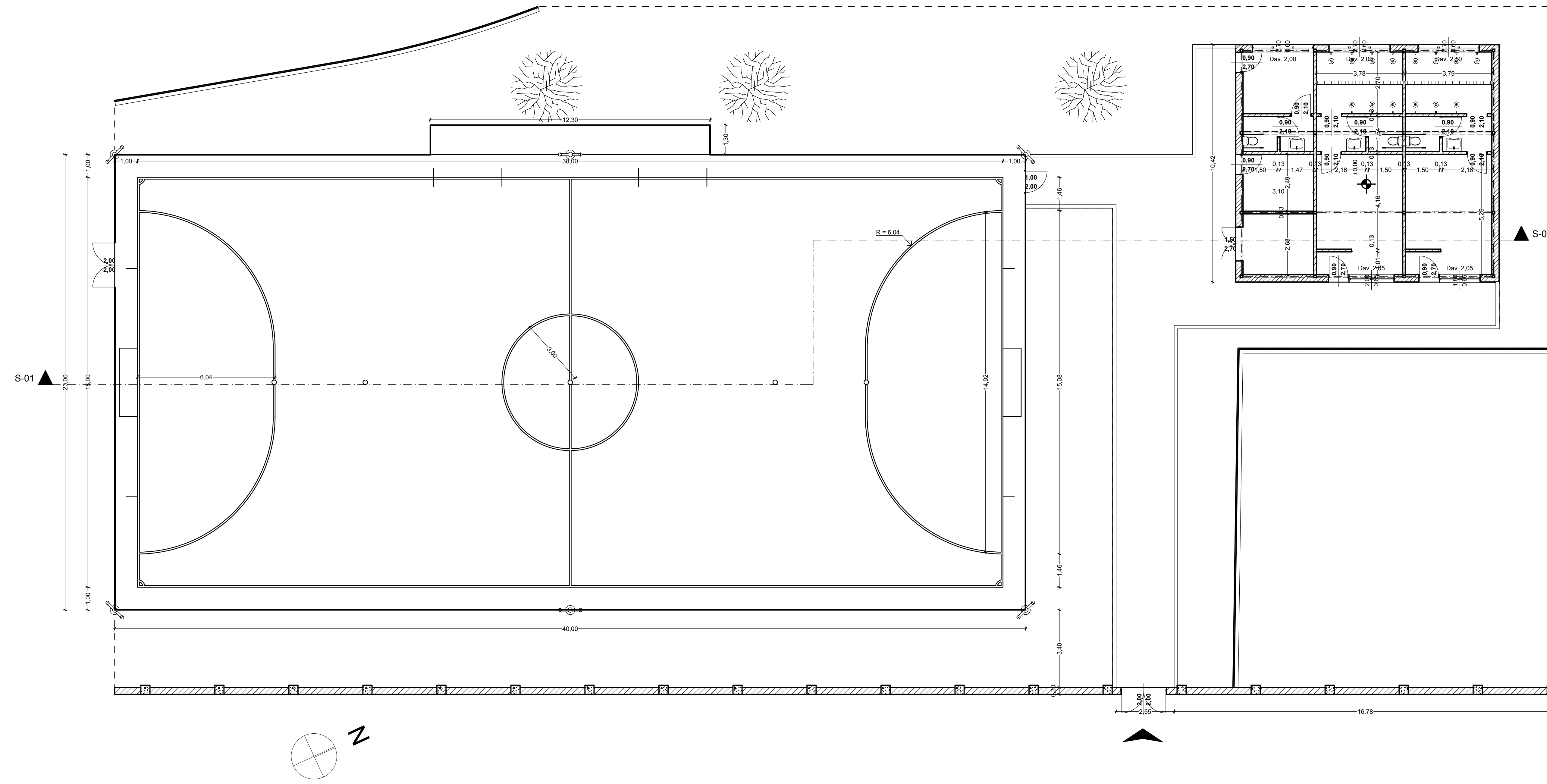
Planimetria piano terra scala 1:100
